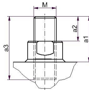
Kolbenstangenende X1 Mit eingesetztem Gewindesttift
